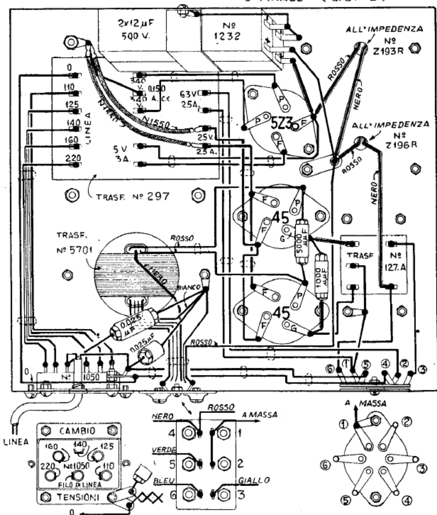
Schema costruttivo. Particolare alimentazione e bassa frequenza.
